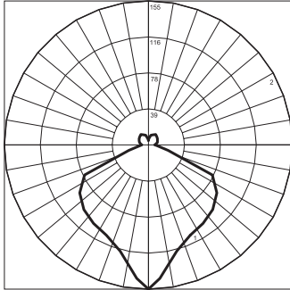
KALEIDOSHADE 2 MINI GLASS SHADE SYL G9 60 WATT HALOGEN LAMP IES Test # K1060QIG
