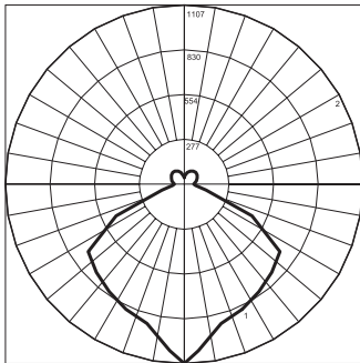
KALEIDOSHADE2 MINI GLASS SHADE SYL CMH70/U/T-4 LAMP IES Test # K1070MAG
