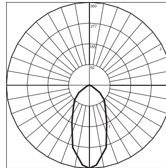
KALEIDOSHADE 2 MINI GLASS SHADE REFLECTOR PHILIPS 70 WATT R-20 LAMP IES Test # K1075RIG
