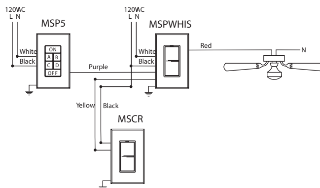
MultiSet Pro Wiring
